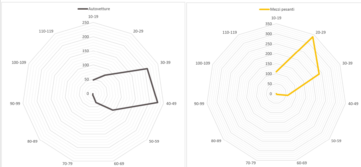
Distribuzione classi di velocità sul totale veicoli giorno
