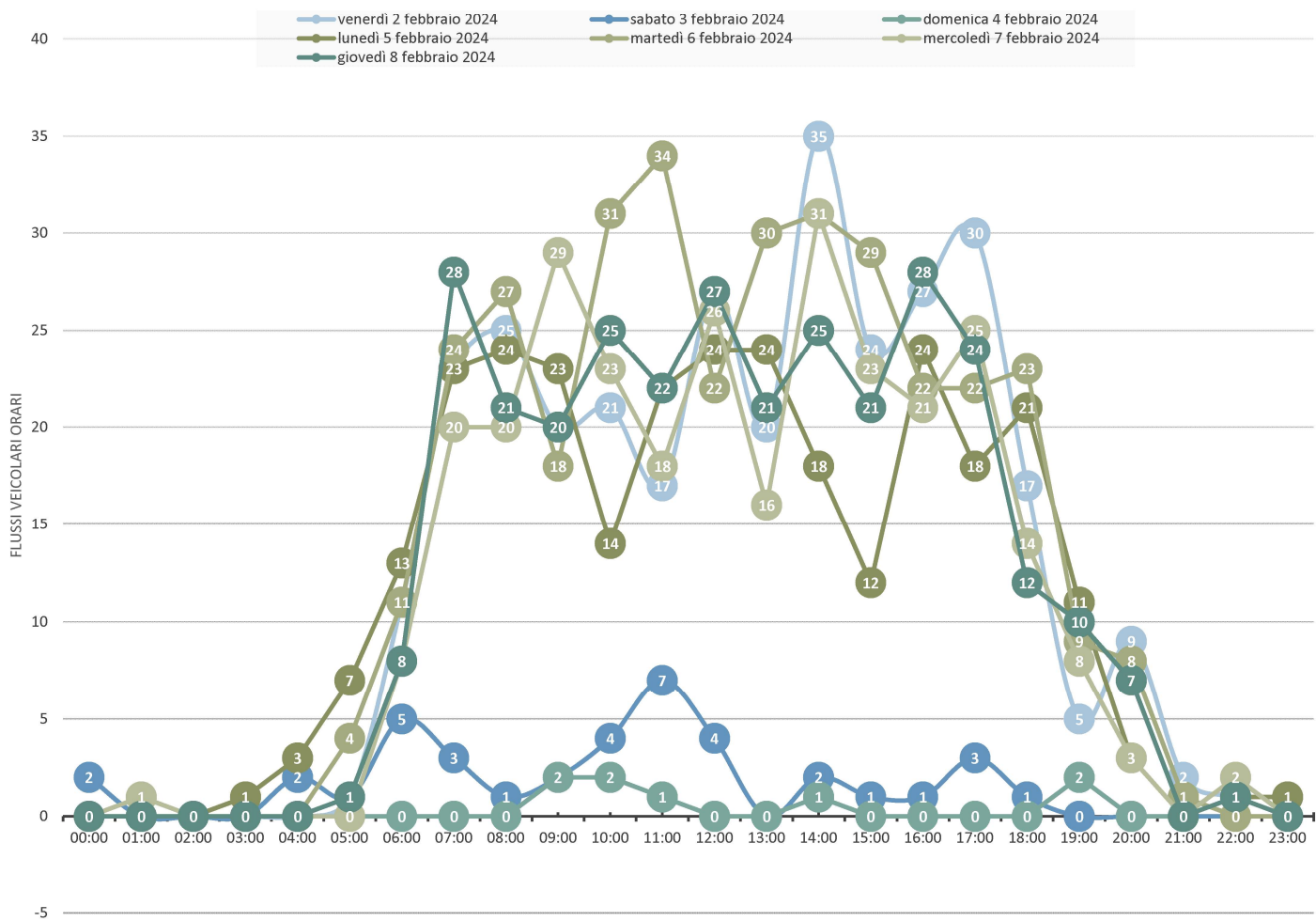
Andamento giornaliero rilievo del traffico SETTIMANA 2 - direzione A+B
