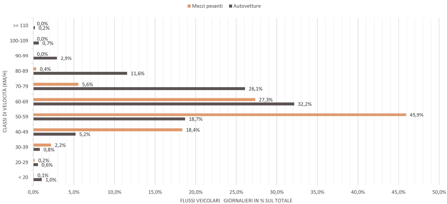
Distribuzione classi di velocità sul totale veicoli giorno
