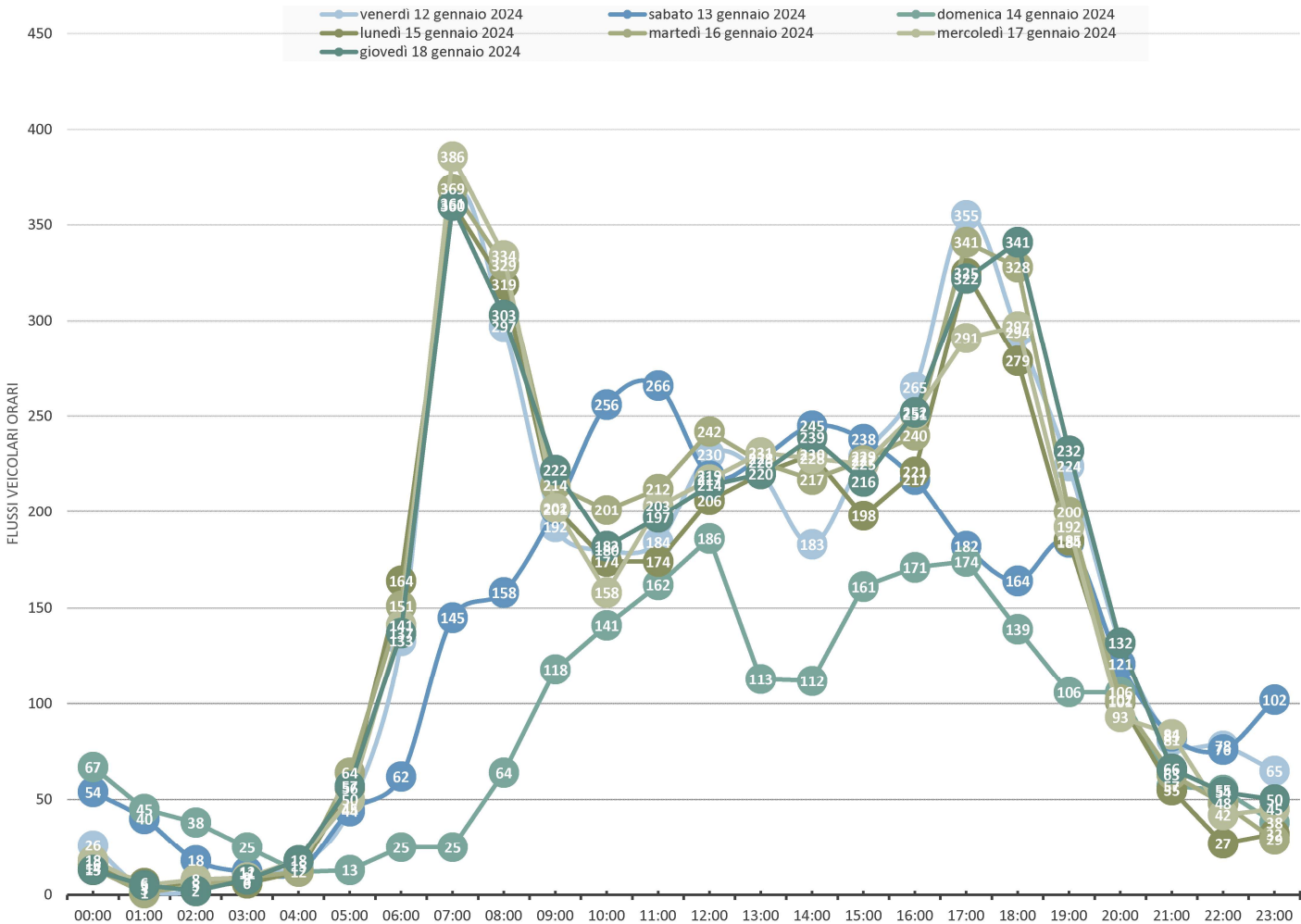
Andamento giornaliero rilievo del traffico SETTIMANA 1 - direzione A+B
