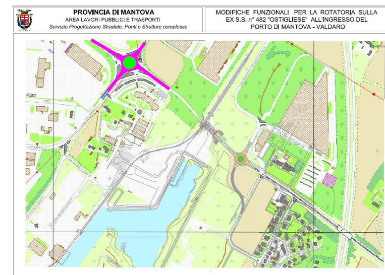
Figura 29. Stralcio planimetrie di progetto adeguamento nodi di connessione esterni al porto. Fonte: Provincia di Mantova.
