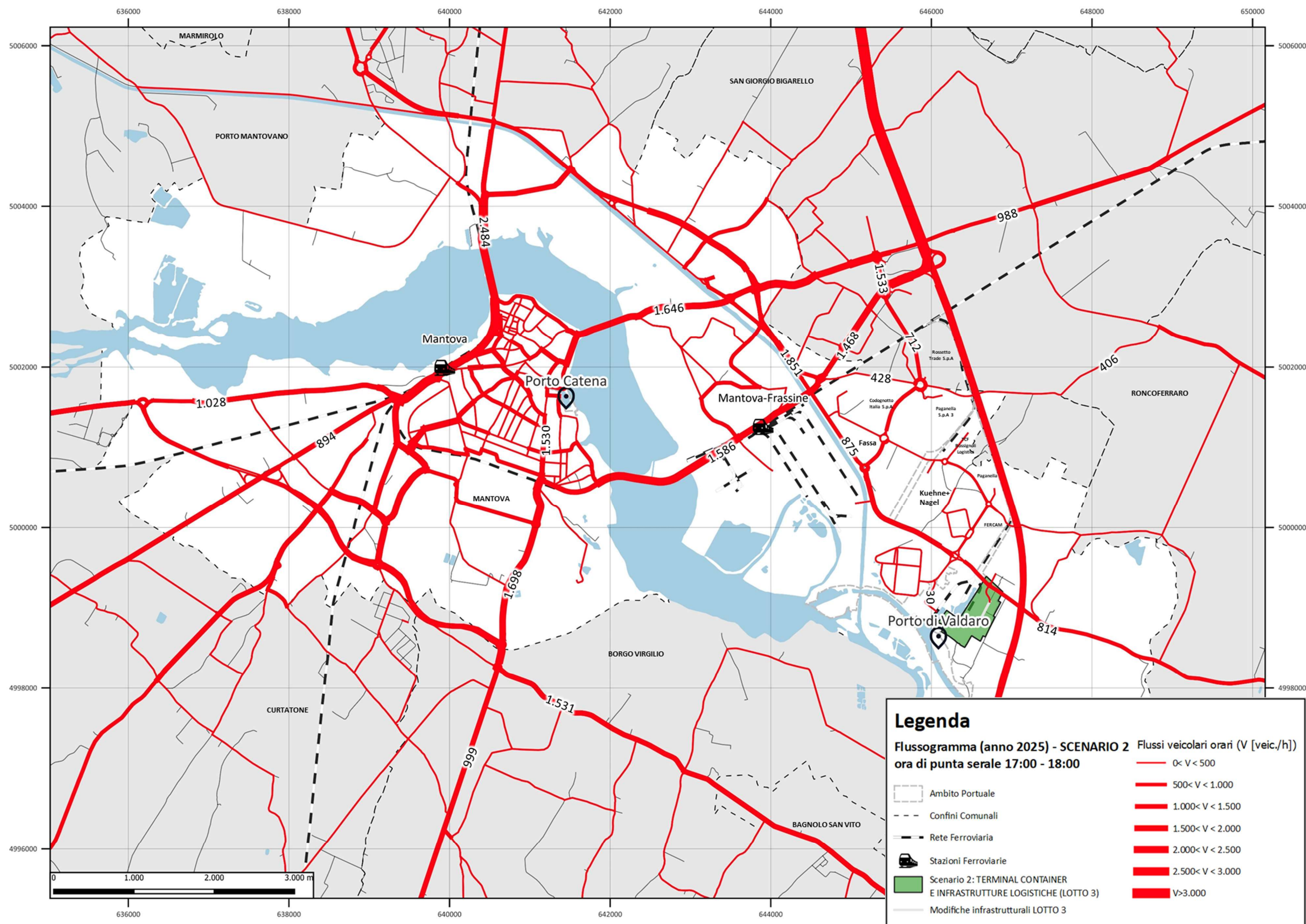
Figura 14. Flussogramma ora di punta - venerdì 17:00-18:00 – SCENARIO 2 – ANNO 2025 – TERMINAL CONTAINER E INFRASTRUTTURE LOGISTICHE - LOTTO 3.
