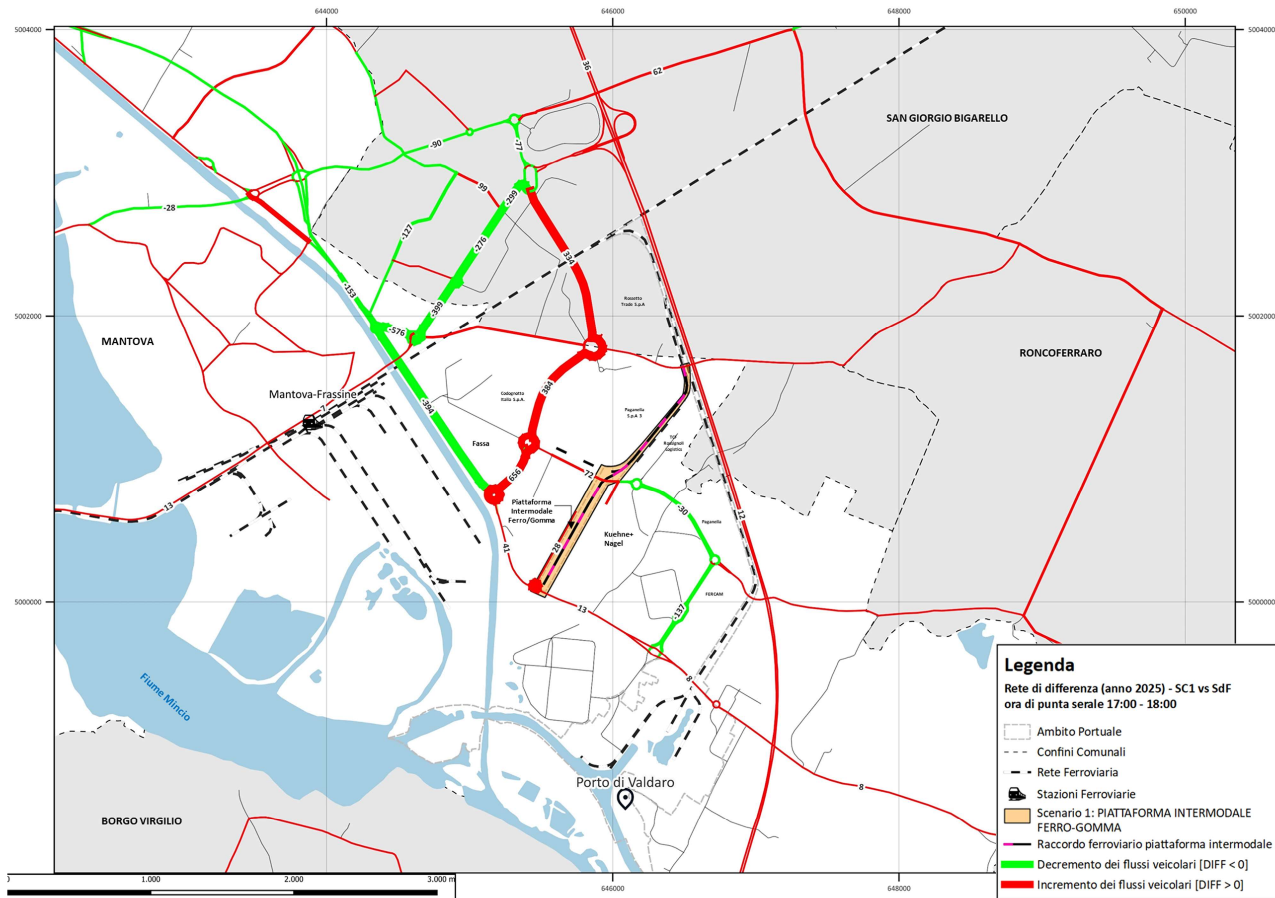
Figura 9. Rete di differenza ora di punta - venerdì 17:00-18:00 – SCENARIO 1 – ANNO 2025 - PIATTAFORMA INTERMODALE FERRO/GOMMA.
