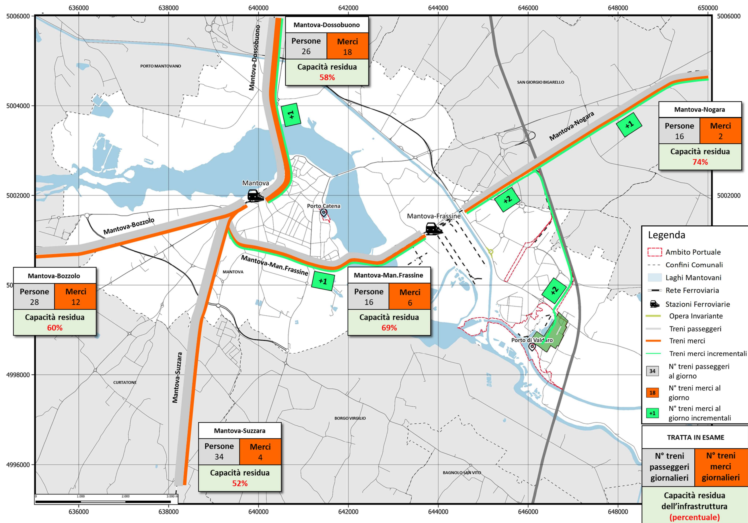
Figura 17. Flussogrammi e capacità residua sull'infrastruttura ferroviaria mantovana – SCENARIO 2 – ANNO 2025 – Terminal container e Infrastrutture logistiche - LOTTO 3.
