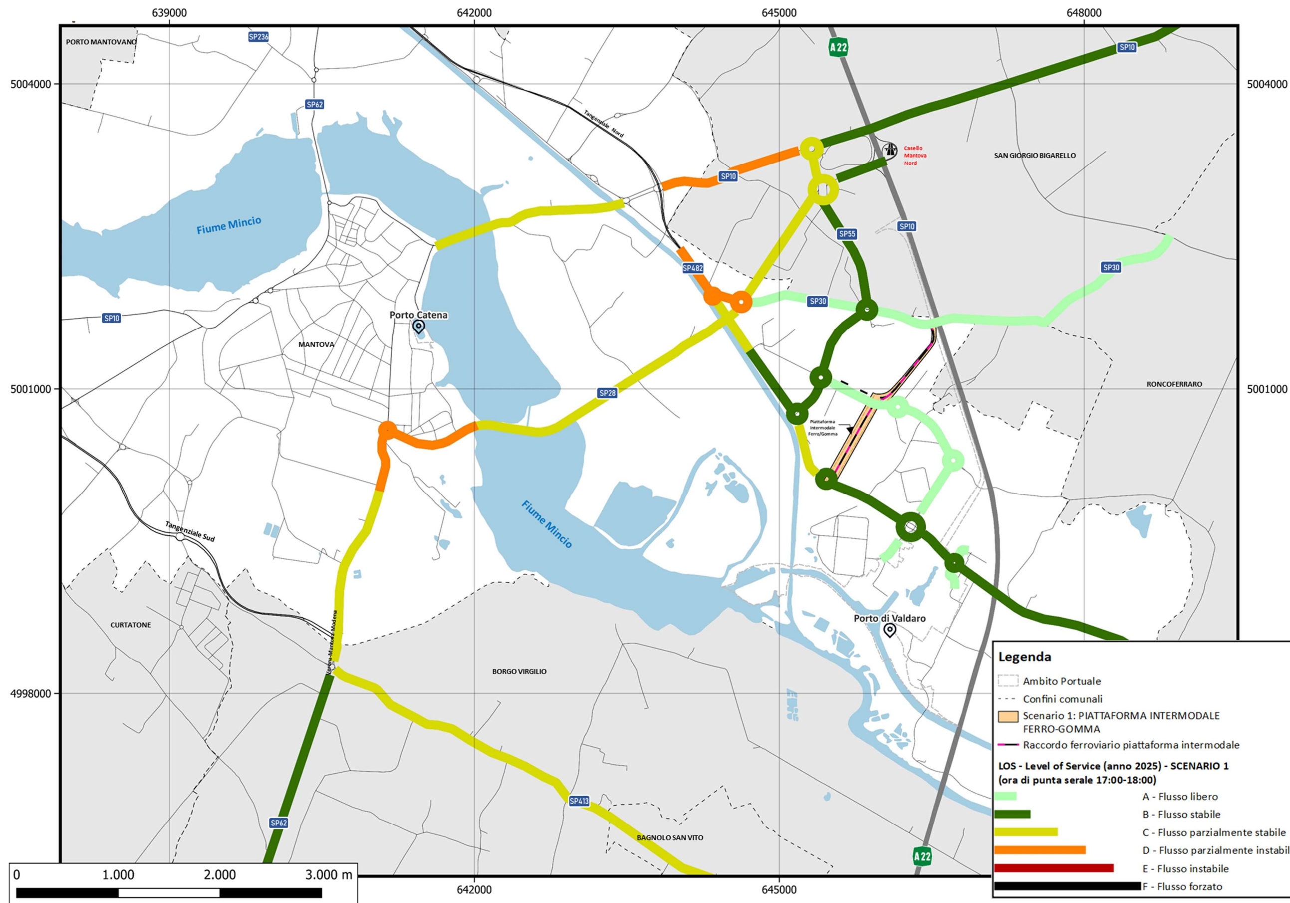
Figura 10. LIVELLI DI SERVIZIO: LOS aste e nodi principali della rete - venerdì 17:00-18:00 – SCENARIO 1 – ANNO 2025 - PIATTAFORMA INTERMODALE FERRO/GOMMA.
