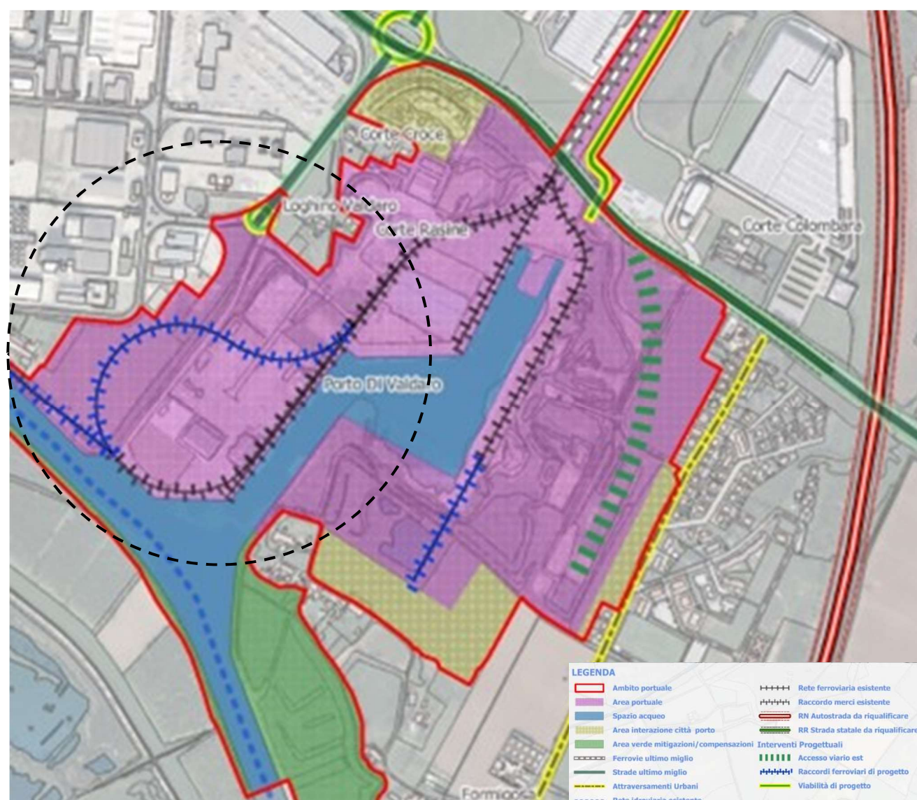
Figura 24. Inquadramento LOTTO 4. Fonte: Provincia di Mantova.
