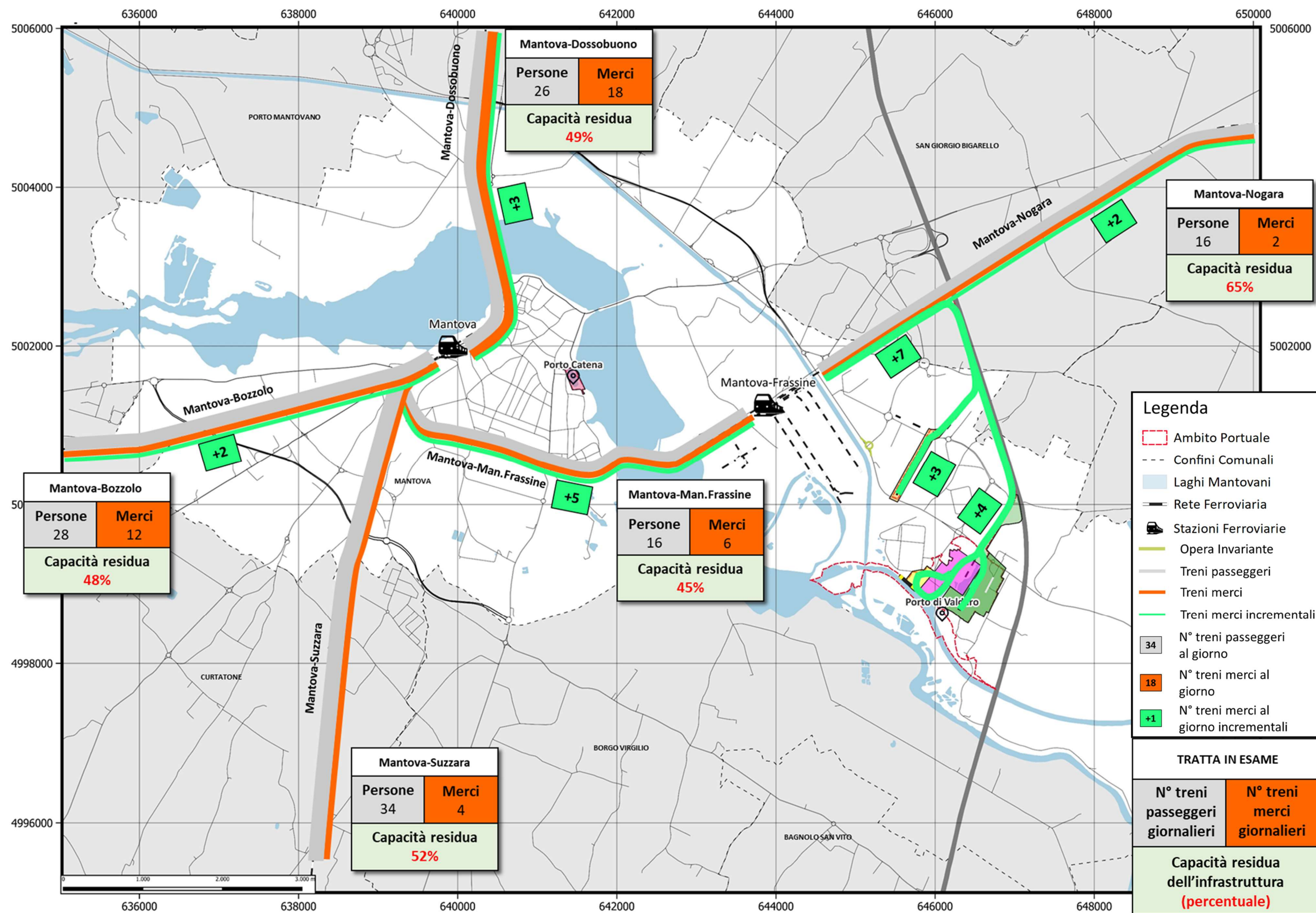
Figura 42. Flussogrammi e capacità residua sull'infrastruttura ferroviaria mantovana – SCENARIO CUMULATO – ANNO 2030.
