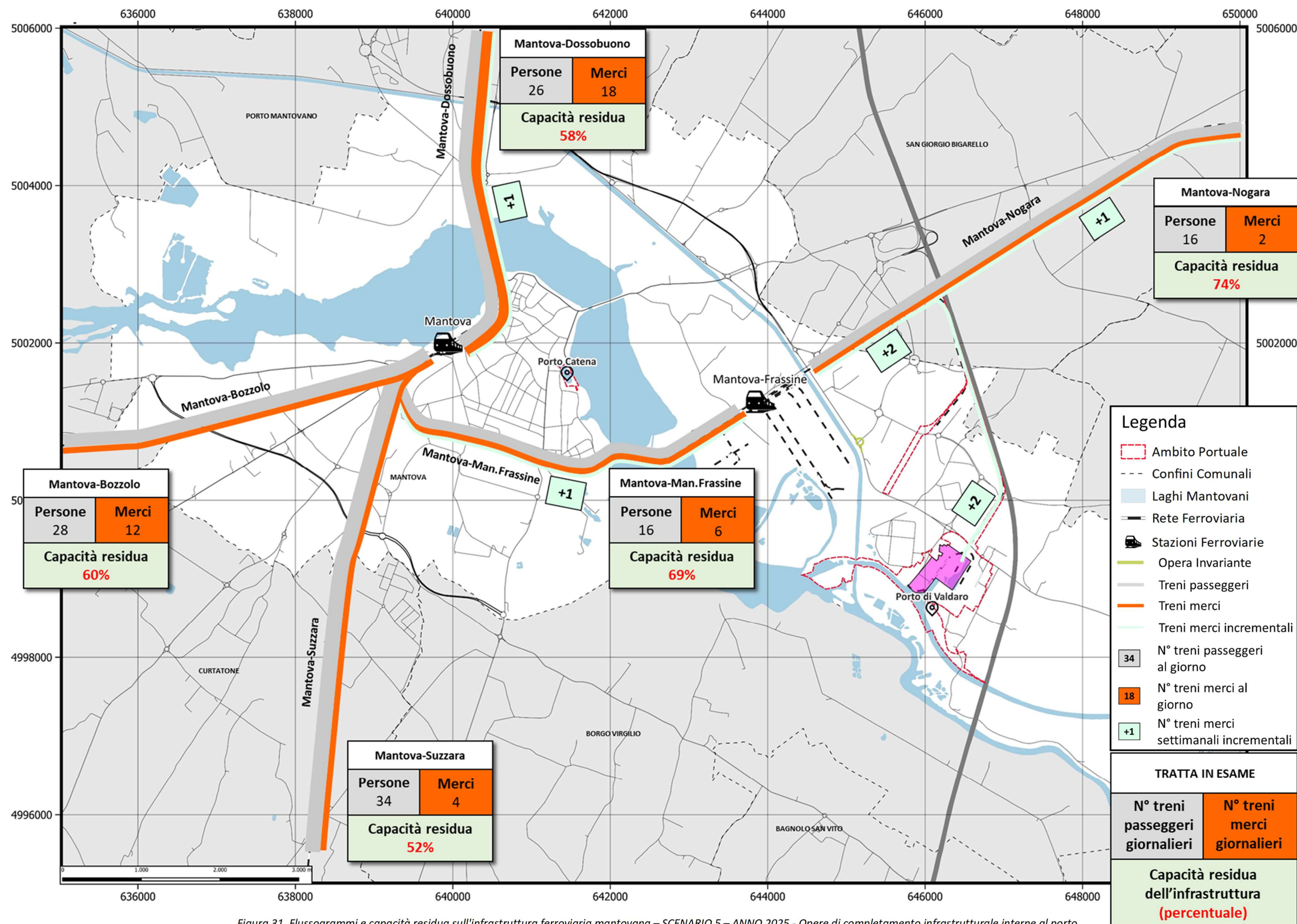
Figura 31. Flussogrammi e capacità residua sull'infrastruttura ferroviaria mantovana – SCENARIO 5 – ANNO 2025 - Opere di completamento infrastrutturale interne al porto.
