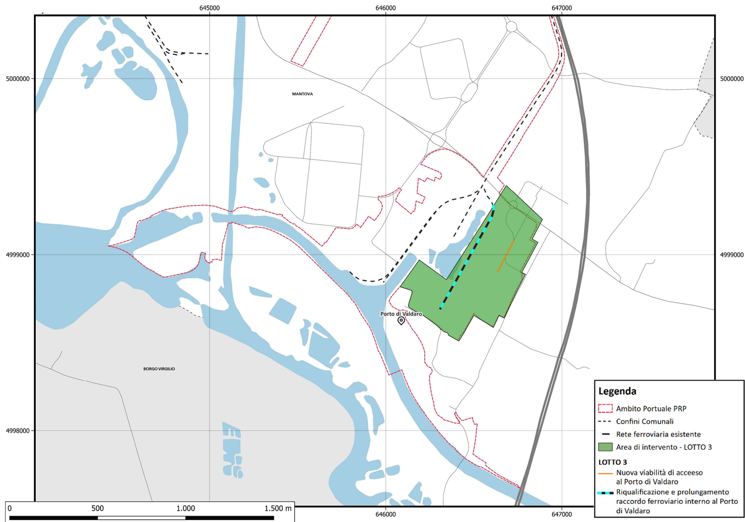
Figura 13. SCENARIO 2: Inquadramento opere infrastrutturali lotto 3.
