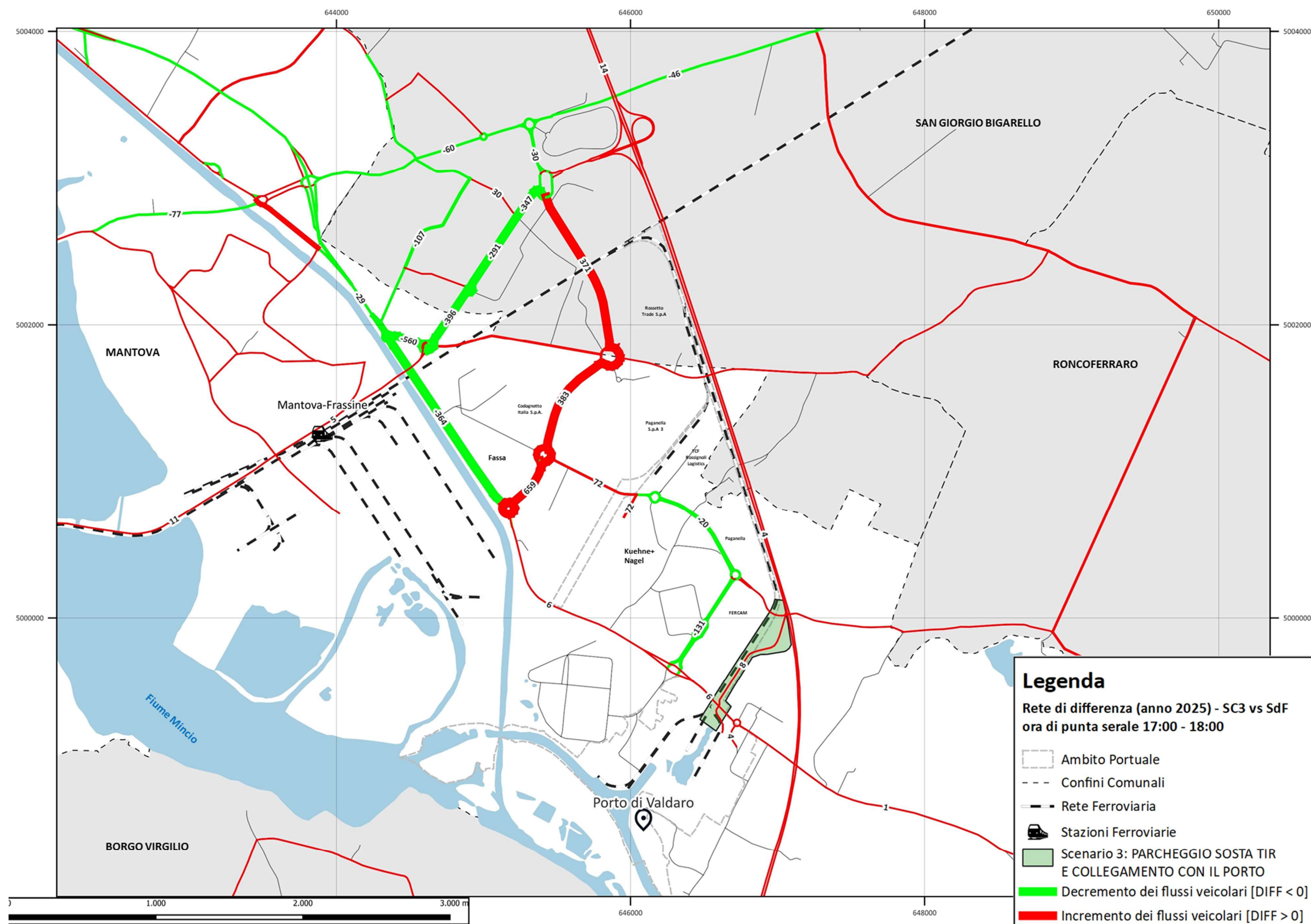
Figura 22. Rete di differenza ora di punta - venerdì 17:00-18:00 – SCENARIO 3 – ANNO 2025 - PARCHEGGIO SOSTA TIR E COLLEGAMENTO CON IL PORTO.
