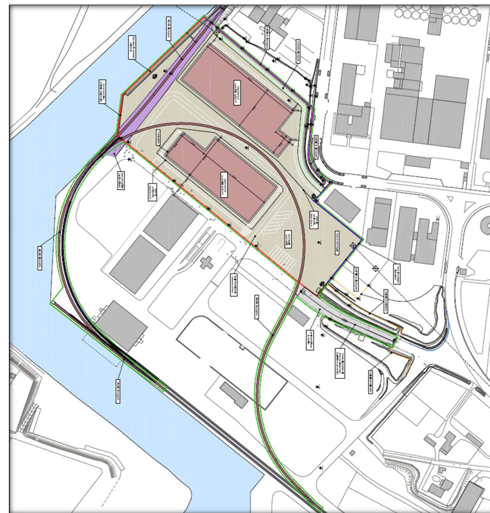
Figura 25. Particolare opere infrastrutturali LOTTO 4. Fonte: Provincia di Mantova.
