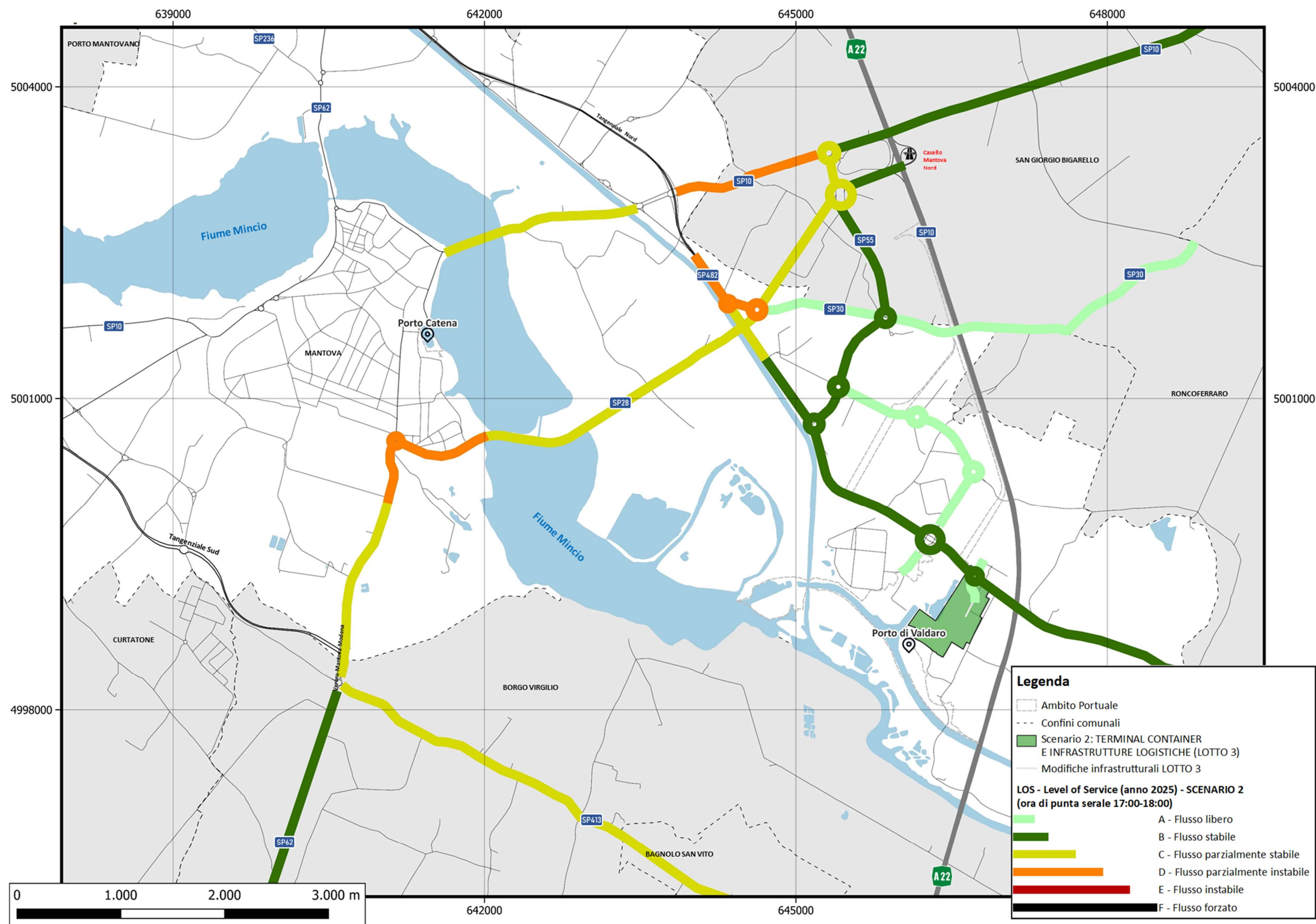
Figura 16. LIVELLI DI SERVIZIO: LOS aste e nodi principali della rete - venerdì 17:00-18:00 – SCENARIO 2 – ANNO 2025 – TERMINAL CONTAINER E INFRASTRUTTURE LOGISTICHE - LOTTO 3.
