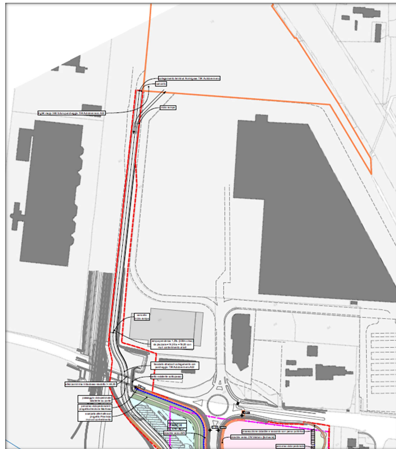
Figura 19. Particolare strada di collegamento parcheggio TIR A22. Fonte: Provincia di Mantova.
