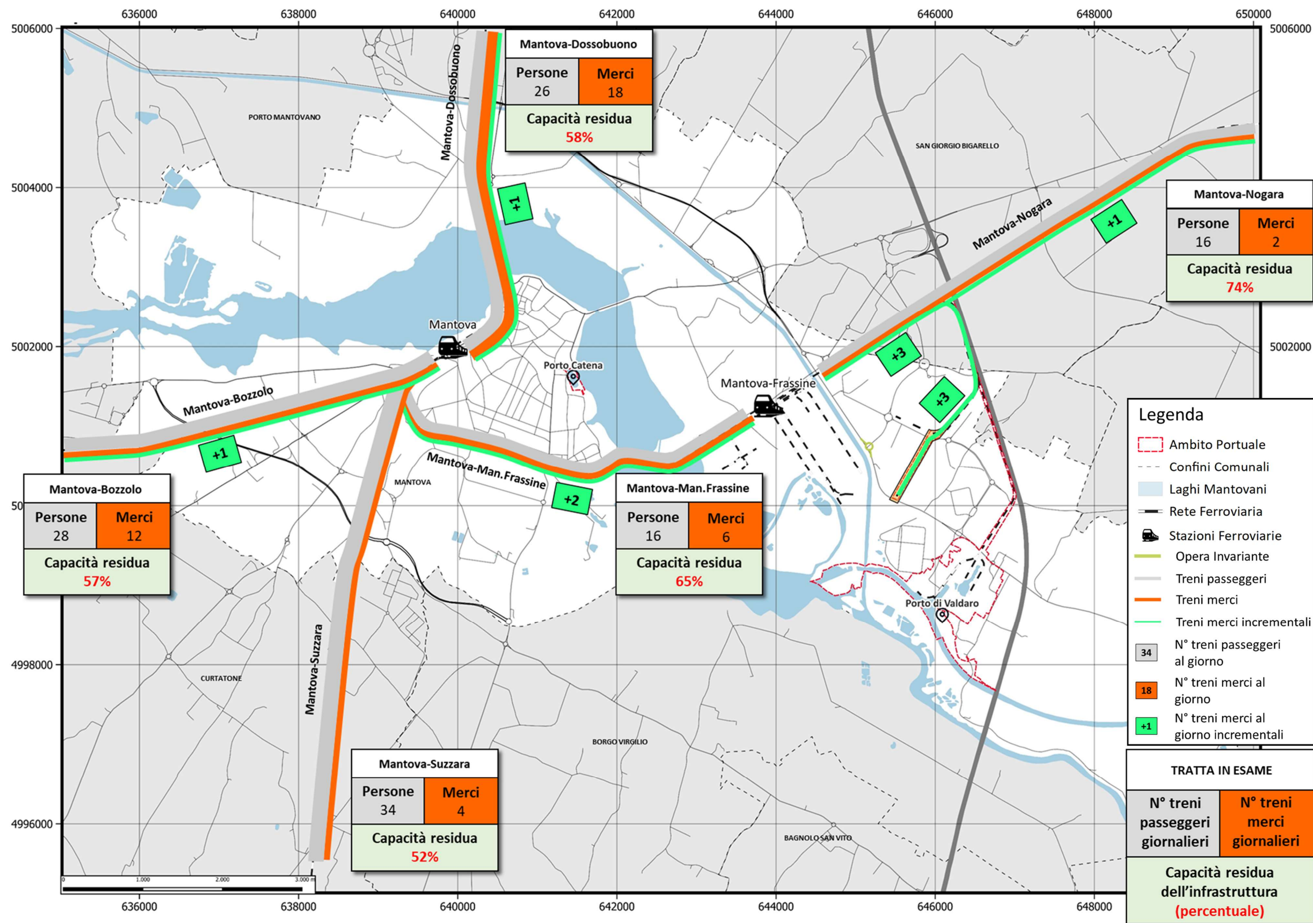
Figura 11. Flussogrammi e capacità residua sull'infrastruttura ferroviaria mantovana – SCENARIO 1 – ANNO 2025 – PIATTAFORMA INTERMODALE FERRO/GOMMA.
