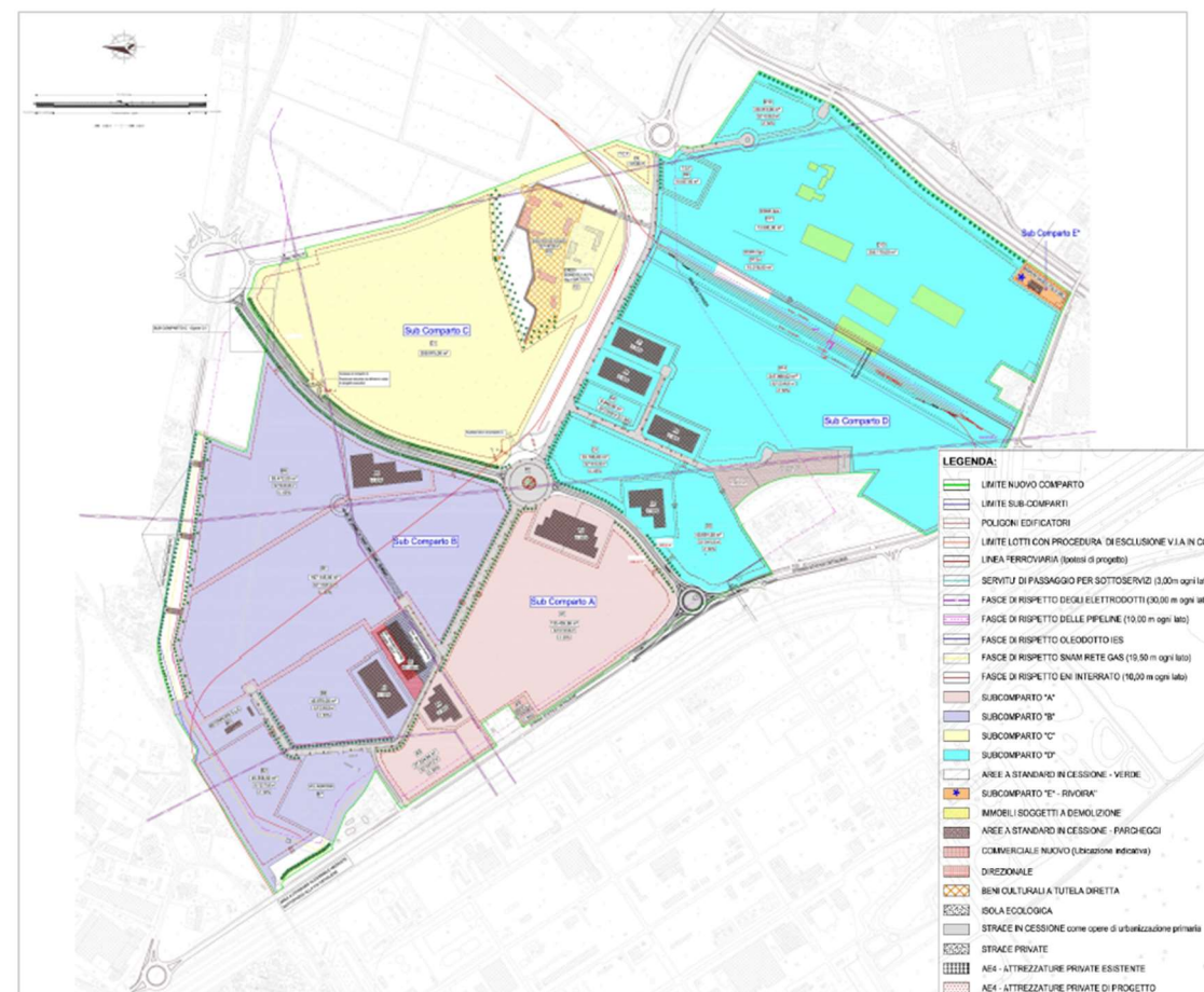
Figura 5. Planimetria di progetto piattaforma intermodale ferro/gomma. Fonte: Provincia di Mantova.
