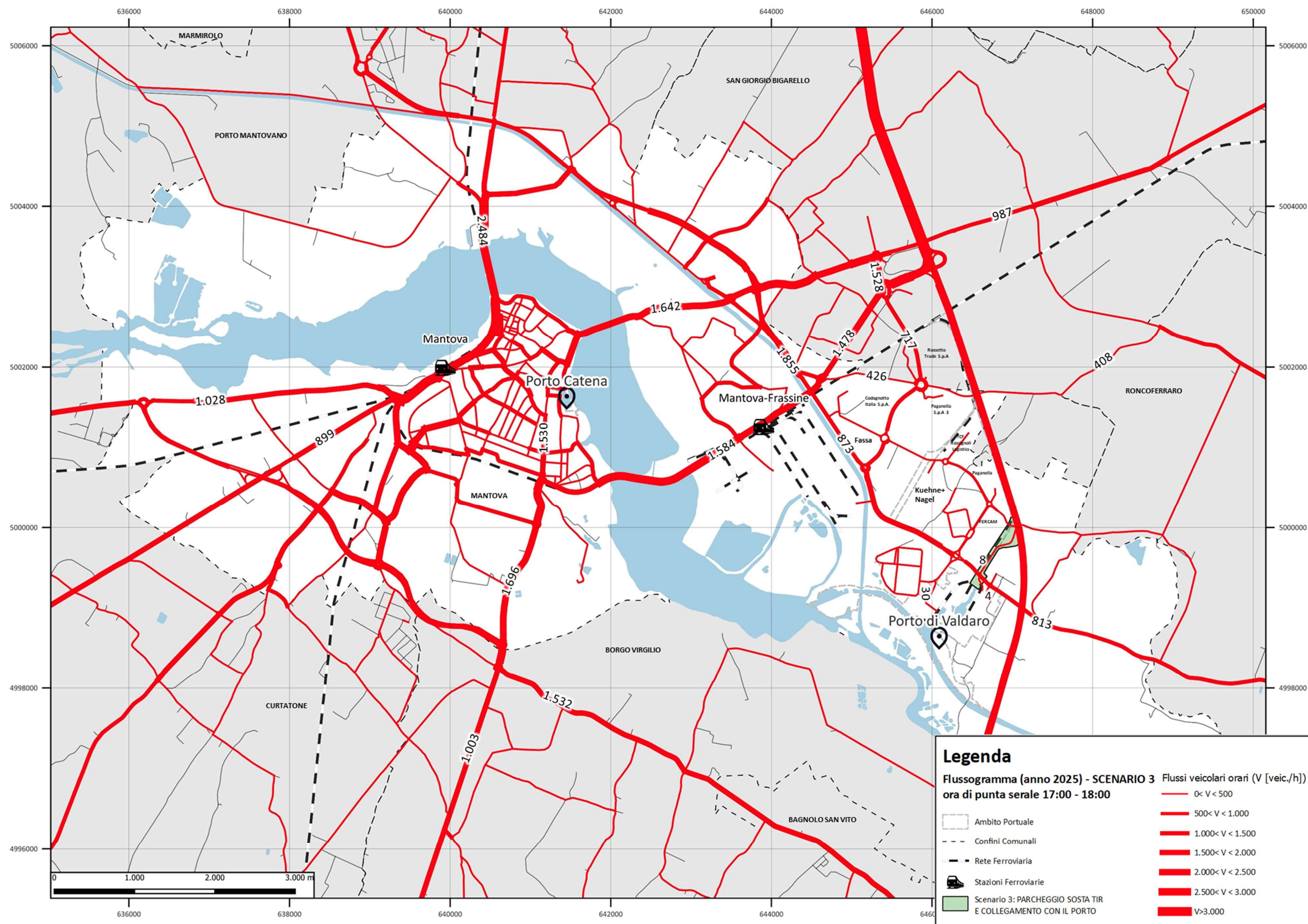
Figura 21. Flussogramma ora di punta - venerdì 17:00-18:00 – SCENARIO 3 – ANNO 2025 - PARCHEGGIO SOSTA TIR E COLLEGAMENTO CON IL PORTO.
