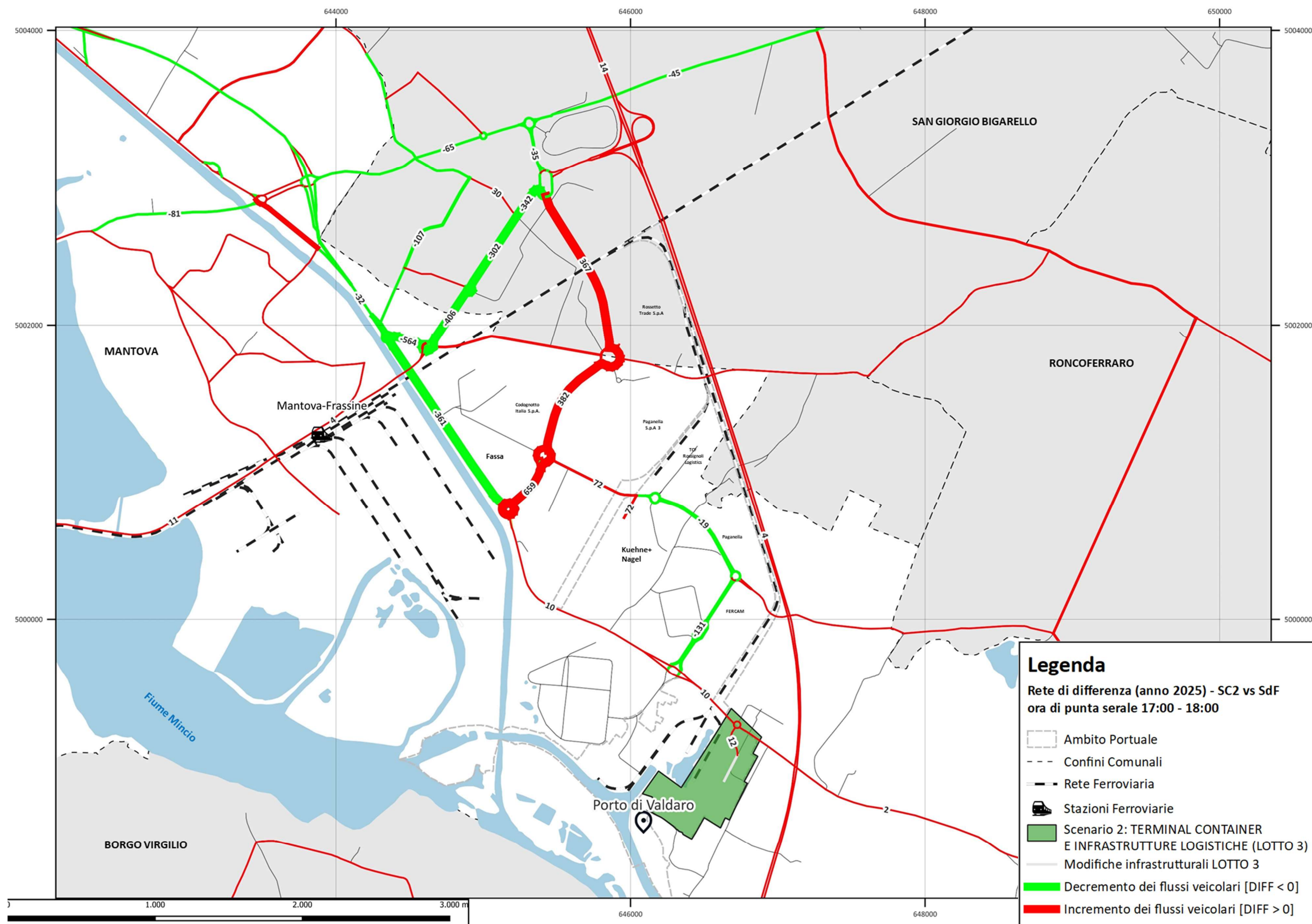
Figura 15. Rete di differenza ora di punta - venerdì 17:00-18:00 – SCENARIO 2 – ANNO 2025 – TERMINAL CONTAINER E INFRASTRUTTURE LOGISTICHE - LOTTO 3.
