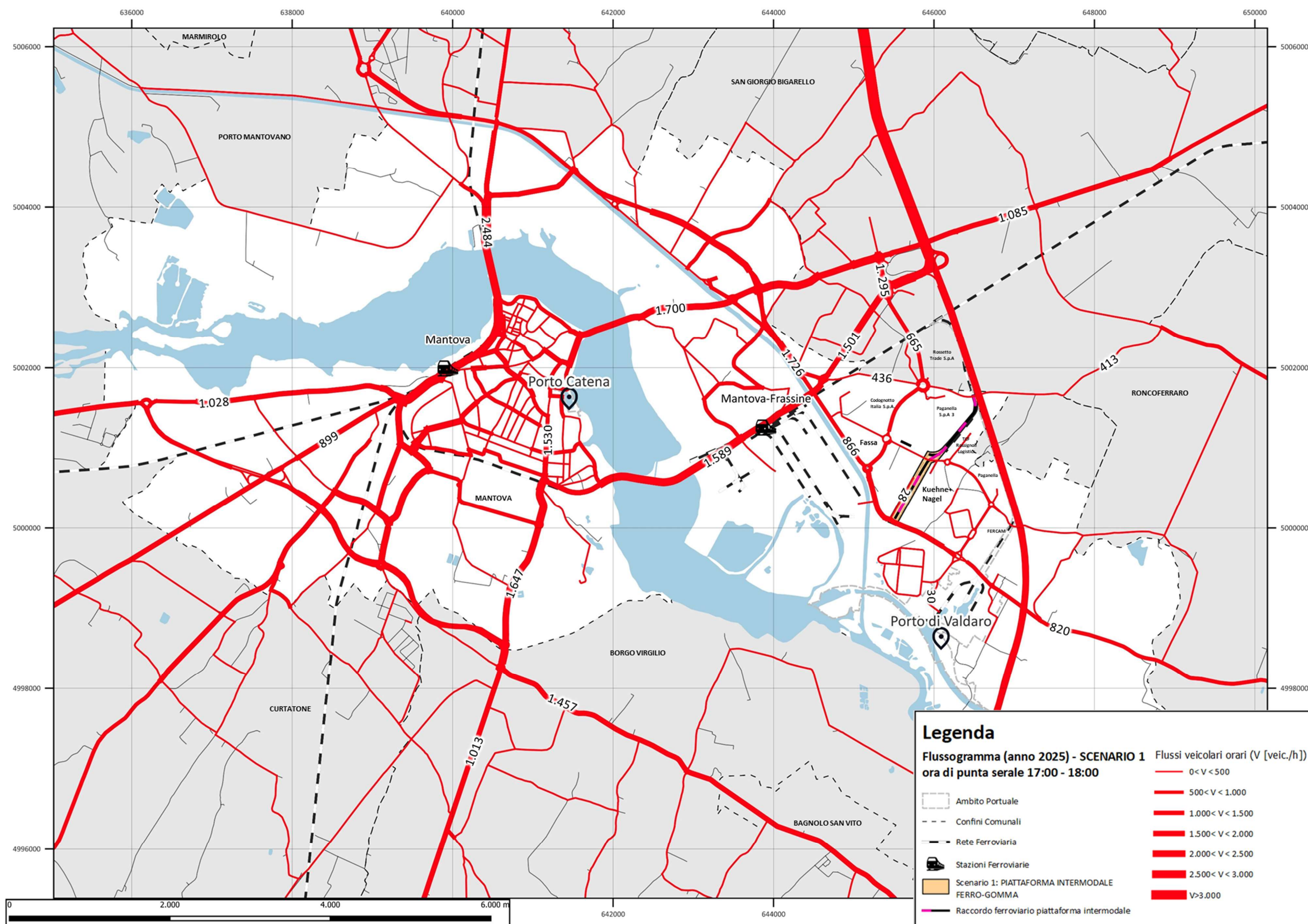
Figura 8. Flussogramma ora di punta - venerdì 17:00-18:00 – SCENARIO 1 – ANNO 2025 - PIATTAFORMA INTERMODALE FERRO/GOMMA.
