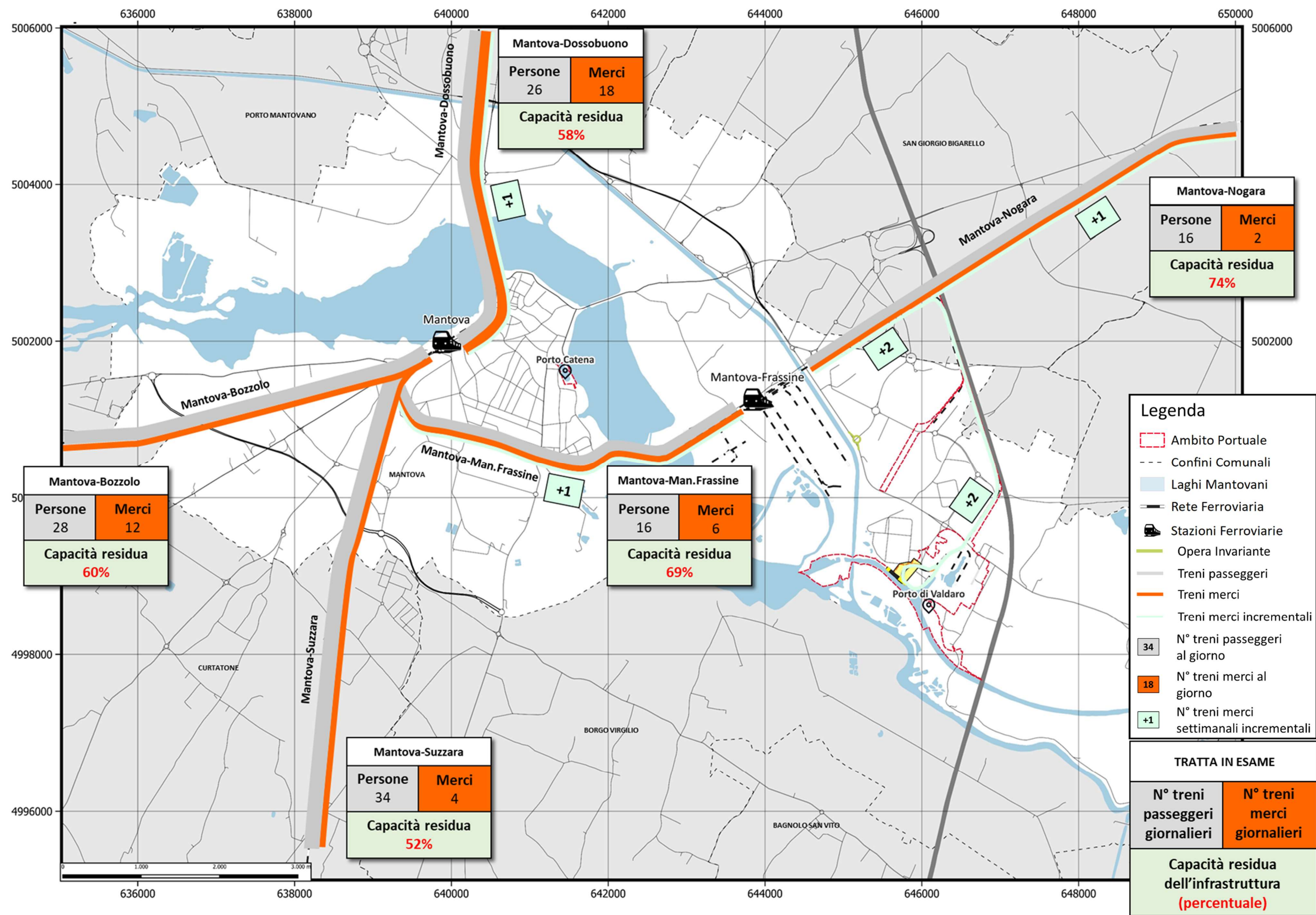
Figura 27. Flussogrammi e capacità residua sull'infrastruttura ferroviaria mantovana – SCENARIO 4 – ANNO 2025 - Prolungamento raccordo ferroviario consorzio agrario nord-est.
