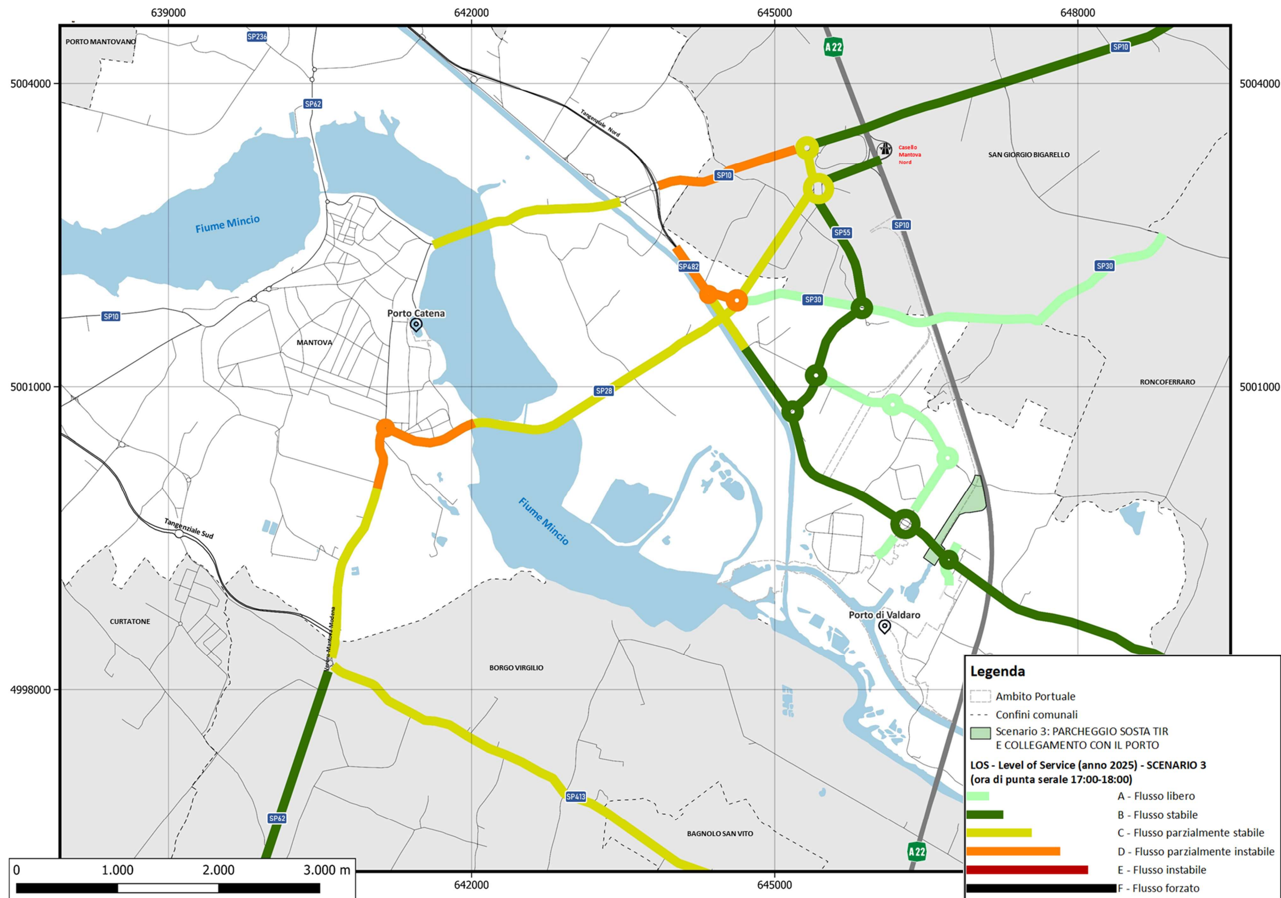
Figura 23. LIVELLI DI SERVIZIO: LOS aste e nodi principali della rete - venerdì 17:00-18:00 – SCENARIO 3 – ANNO 2025 - PARCHEGGIO SOSTA TIR E COLLEGAMENTO CON IL PORTO.
