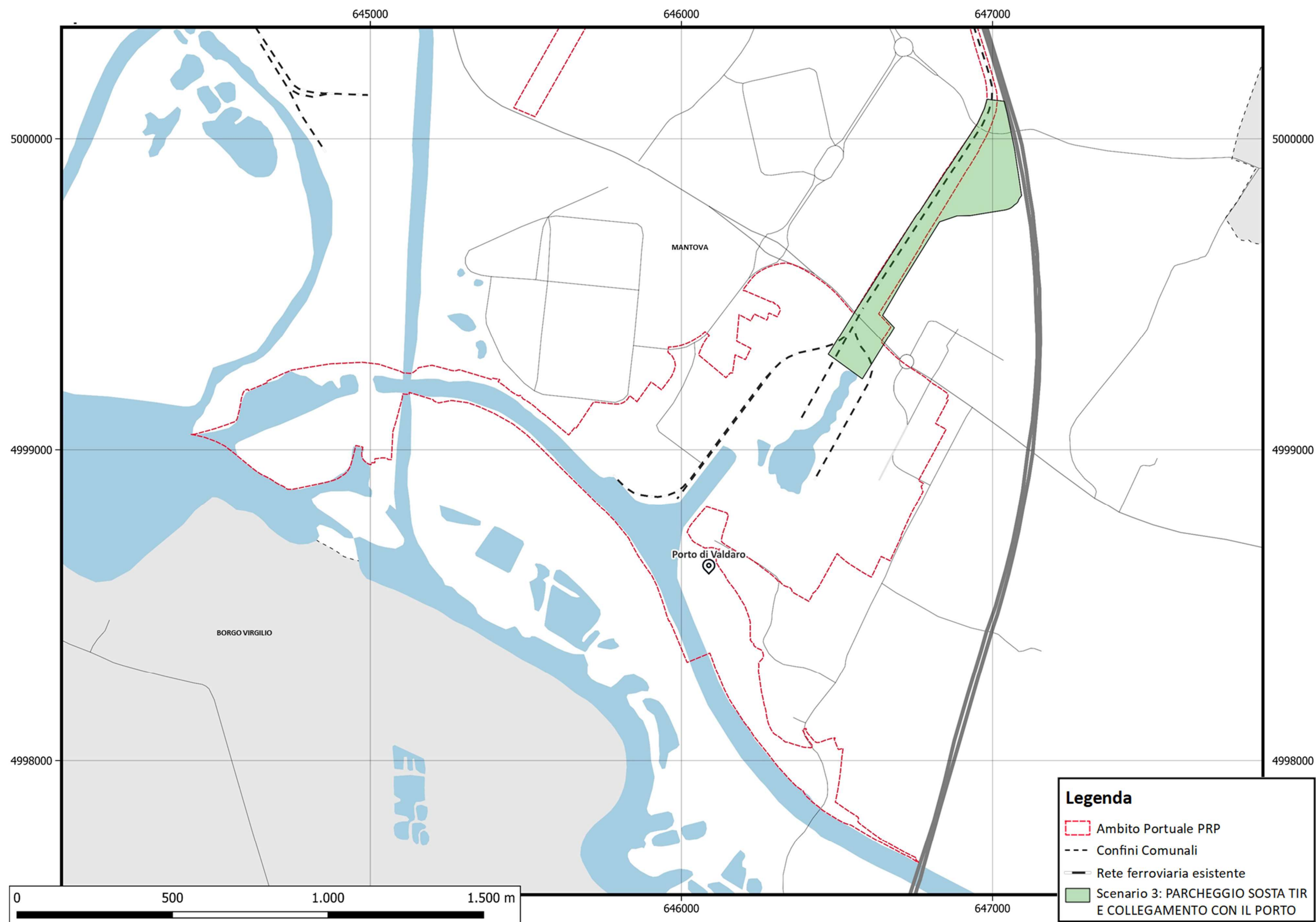
Figura 20. SCENARIO 3: Inquadramento opere infrastrutturali di collegamento tra il Porto di Valdaro e il parcheggio TIR A22.
