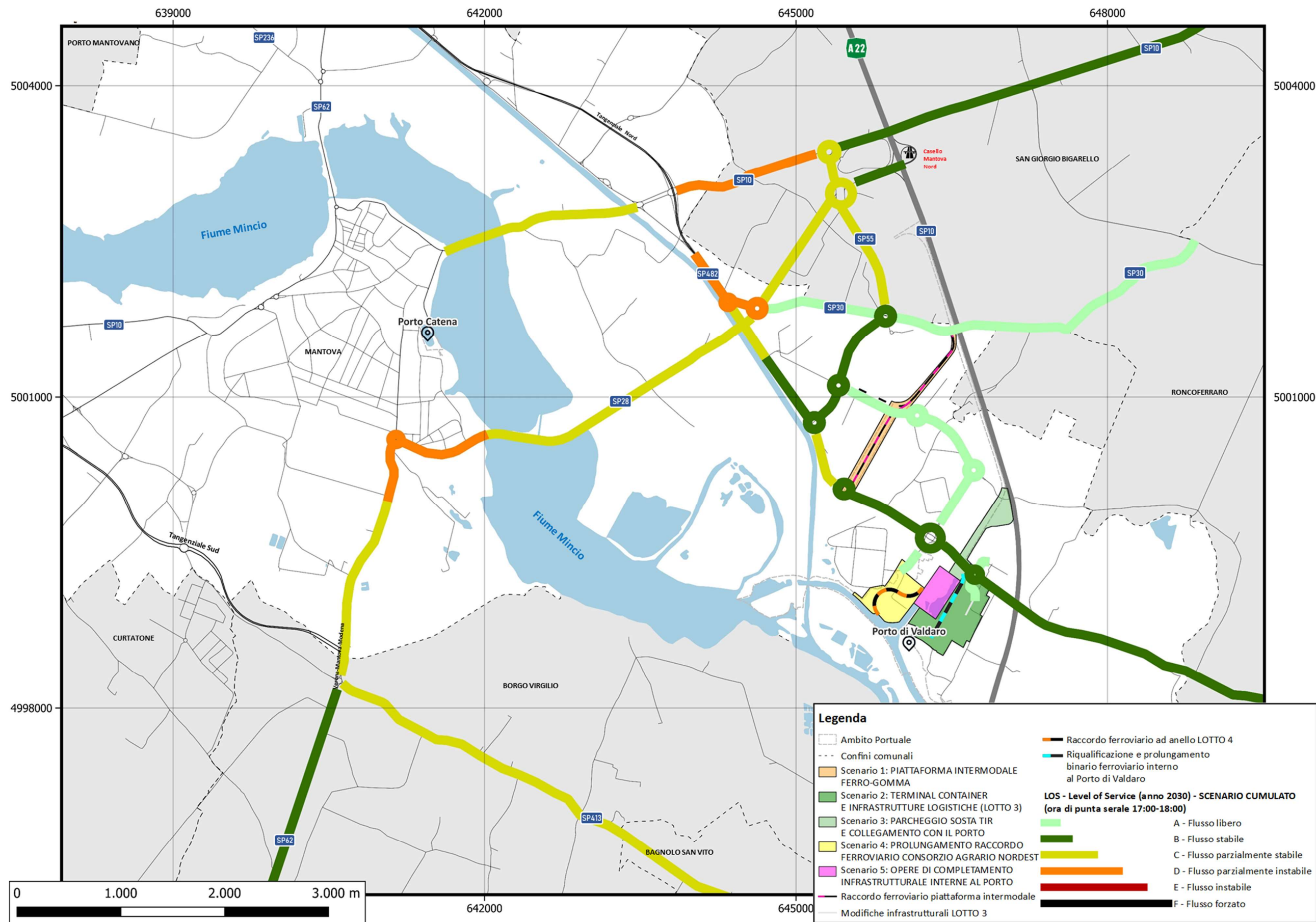
Figura 41. LIVELLI DI SERVIZIO: LOS aste e nodi principali della rete - venerdì 17:00-18:00 – SCENARIO CUMULATO – ANNO 2030.
