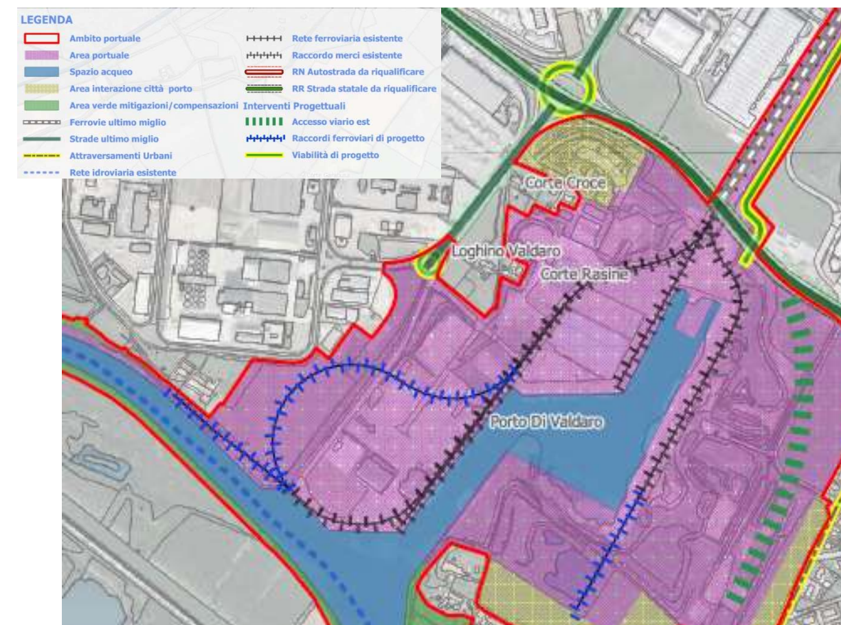
Figura 12. Lotto 3: individuazioni delle opere in progetto.
