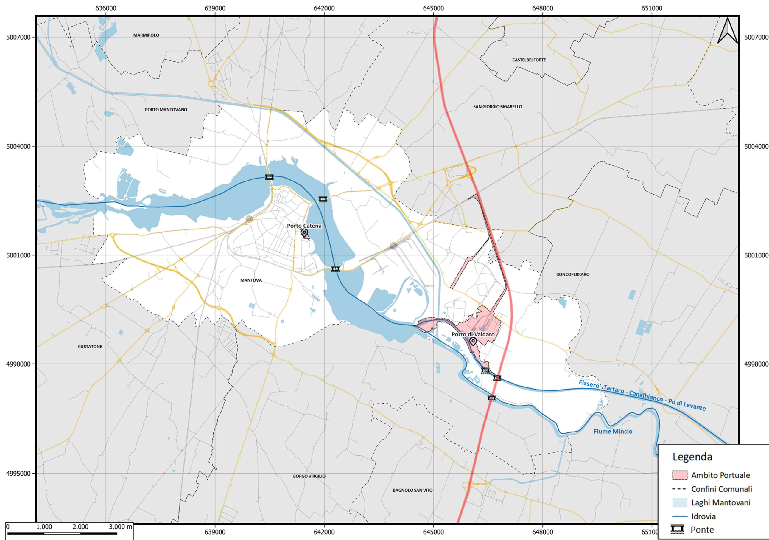
Figura 42. Interferenze tra rete idroviaria e viabilità ordinaria.
