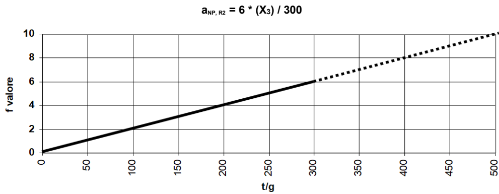
Grafico 2 - a NP,R2 - funzione valore (a RANK ) relativa alla coppia di indicatori X 1 = Rifiuti non pericolosi, X 2 = R2
