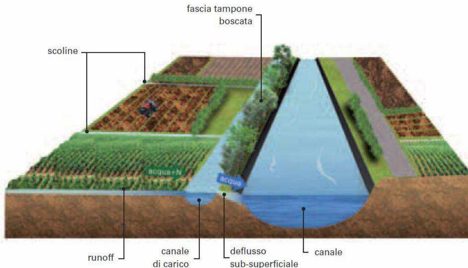
Figura 3.2 – Schema progettuale di una fascia tampone con canale di carico per il trattamento dei carichi di azoto (N) e fosforo (P) veicolati tramite deflusso sub-superficiale e runoff.
